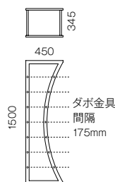
図面はYT-26/27共通です。
