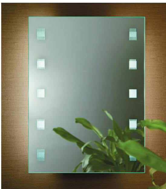
LM-901-EN (昼白色)・LM-901-EL (電球色) ■ W450×H900×厚55mm / 12.5kg ■ ミラー(エッチング)・スチール ■ 蛍光灯 18w×2 / 消費電力46w / インバータ ¥129,150 (本体価格 ¥123,000)
